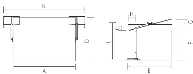
FLEXY MIT ALUMINIUMFUSS
