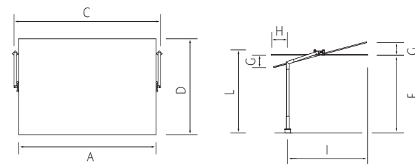
FLEXY MIT AUFSATZ AUF BODENHÜLSE
